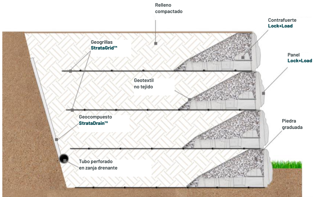
El sistema completo: módulo Lock+Load, geogrilla StrataGrid™, geotextil de separación, geocompuesto StrataDrain™ y dren de pie
